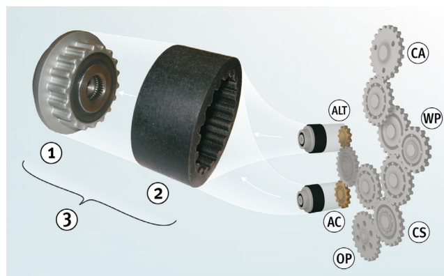
Bild 1: eneratorfrinav med flexibel kopplingsmuff och drivning genom främre kugghjul.
