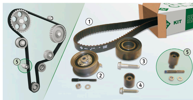
Obrázek 1: Schéma pohonu 1.9 TDI/SDI a obsah balení KIT 530 0361 10/530
