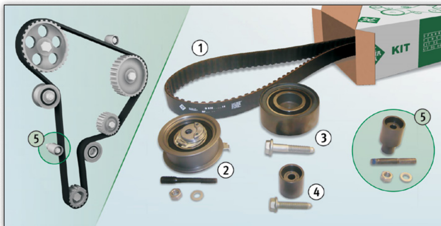
Fig. 1: Esquema de transmisión 1.9 TDI/SDI y contenido del KIT 530 0361 10/530 0082 10
