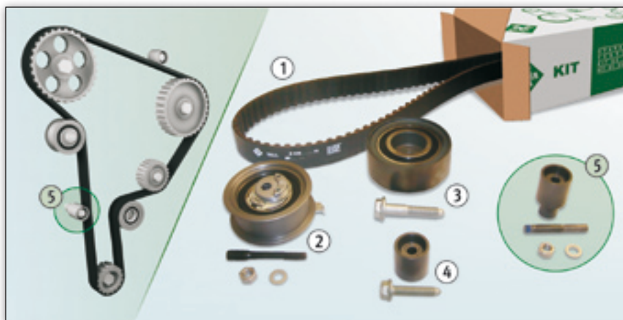
Fig. 1: Aandrijfschema 1.9 TDI/SDI en verpakking inhoud KIT 530 0361 10/530 0082 10
