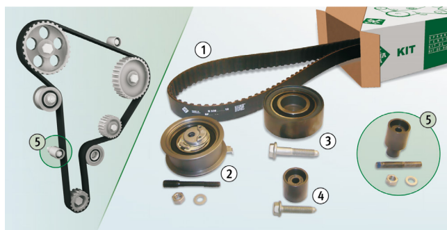
Figur 1: Drev-diagram 1.9 TDI/SDI og pakkeinnhold for SETT 530 0361 10/530 0082 10
