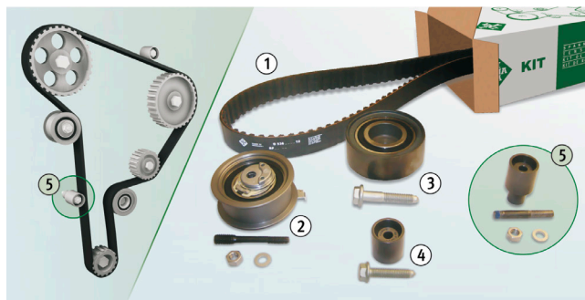
Figura 1: Diagramă distribuție 1,9 TDI/SDI și conținutul pachetului pentru KIT-urile 530 0361 10/530 0082 10
