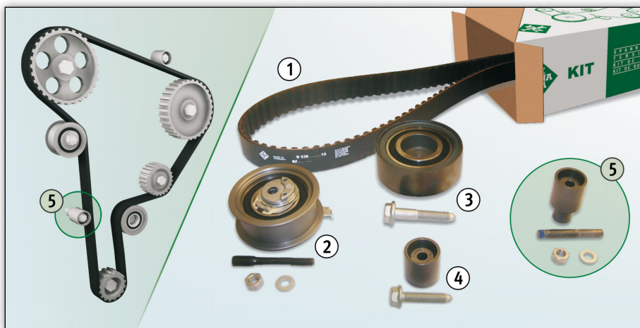
Obrázok 1: Schéma pohonu 1.9 TDI/SDI a obsah balenia KIT 530 0361 10/530 0082 10
