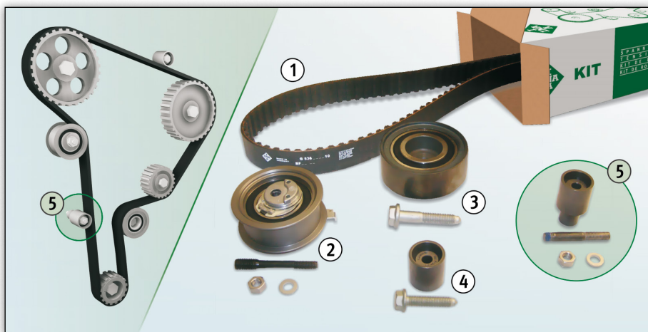
Slika 1: ogonska shema 1.9 TDI/SDI in vsebina garniture 530 0361 10/530 0082 10
