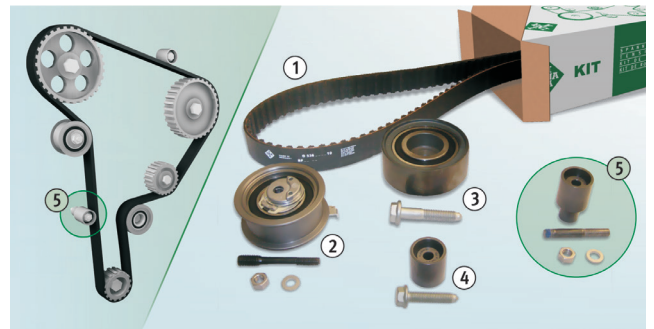
Зображення 1: Схема приводу ГРМ двигунів 1.9 TDI/SDI і вміст комплекту 530 0361 10/530 0082 10
