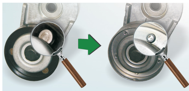
Figur 1: Detaljert visning over rullen i den tidligere utformingen (venstre) og nye utformingen (høyre)
