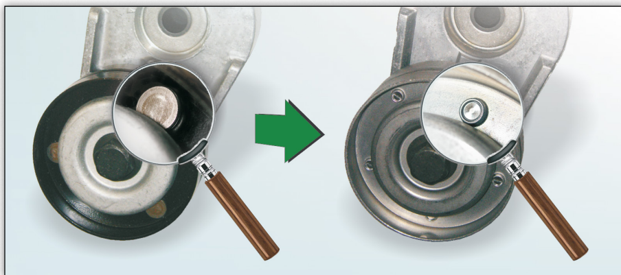
Obrázok 1: Detailný pohľad na vodiace kladky v doterajšom vyhotovení (vľavo) a v novom vyhotovení (vpravo)
