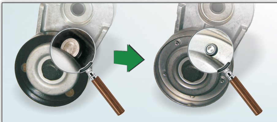
Slika 1: Natančen prikaz valjev v dosedanji izvedbi (levo) in novi izvedbi (desno)
