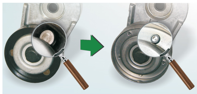
Obrázek 1: Detailní pohled na vodící kladky v dosavadním provedení (vlevo) a v novém provedení (vpravo)
