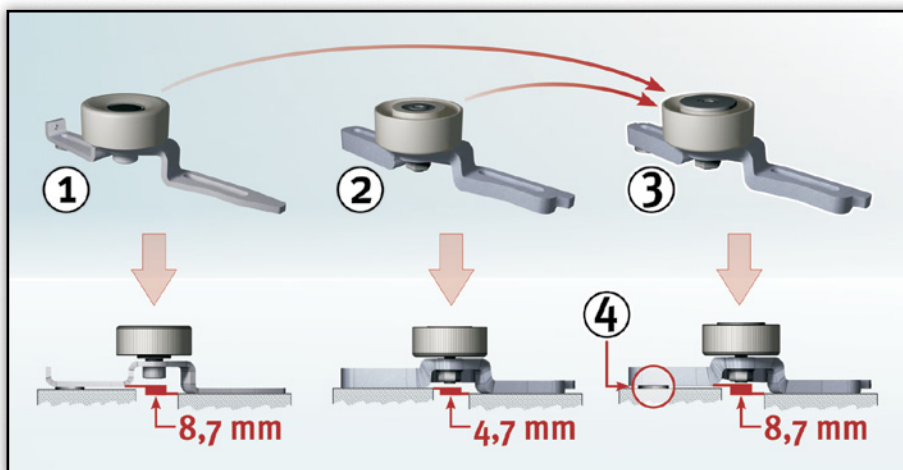
Figura 1: Raffigurazione dei singoli rulli tenditori con le loro differenze
