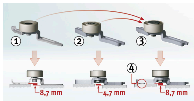
Figura 1: Role întinzătoare și diferențele dintre acestea
