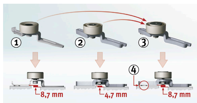
Рисунок 1: Иллюстрация натяжных роликов и их разница
