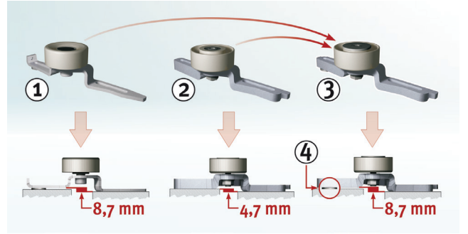
Şekil 1: Aynı gergi kasnaklarının ve bunların farklılıklarının gösterimi
