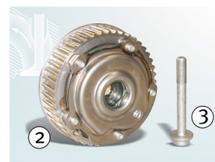
Obrázek 2: Seřízení vačkové hřídele na straně výfuku 427 1005 10 a centrální šroub 41301*
