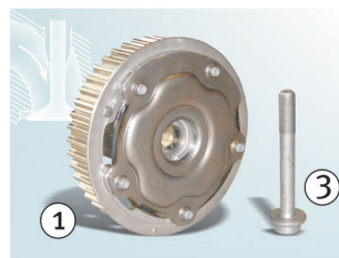
1. ábra: Szívóoldali vezérműtengely-állító 427 1004 10 és központi csavar 41301*
