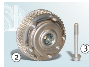
2. ábra: Kipufogó oldali vezérműtengely-állító 427 1005 10 és központi csavar 41301*
