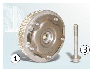
Figura 1: Unitate de fazare dinspre admisie 427 1004 10 și șurub central 41301*
