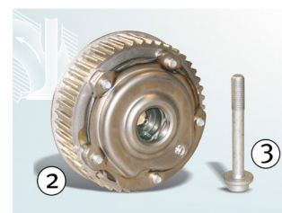
Рисунок 2: Регулятор фаз газораспределения на выпуск 427 1005 10 и центральный болт 41301*
