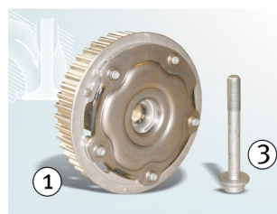
Рисунок 1: Регулятор фаз газораспределения на впуск 427 1004 10 и центральный болт 41301*
