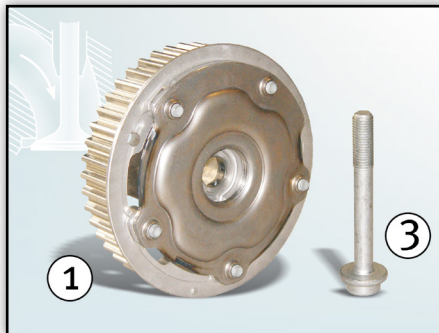
Slika 1: Fazna enota odmikalne gredi za sesalno stran 427 1004 10 in sredinski vijak 41301*
