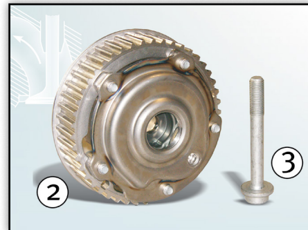
Slika 2: Fazna enota odmikalne gredi za izpušno stran 427 1005 10 in sredinski vijak 41301*
