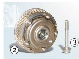
Bild 2: Kamaxeljustering avgassida 427 1005 10 och centralskruv 41301*
