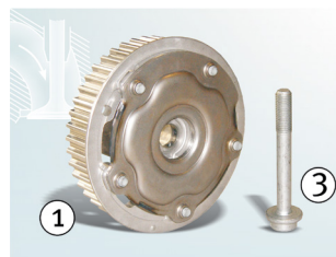
Bild 1: Kamaxeljustering insugsida 427 1004 10 och centralskruv 41301*
