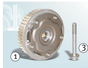
Зображення 1: Регулятор фаз газорозподілу з боку впуску 427 1004 10 і центральний гвинт 41301*
