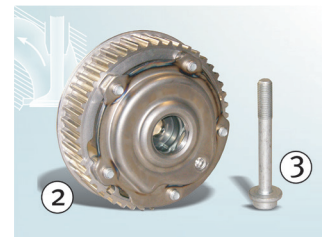
Зображення 2: Регулятор фаз газорозподілу з боку випуску 427 1005 10 і центральний гвинт 41301*
