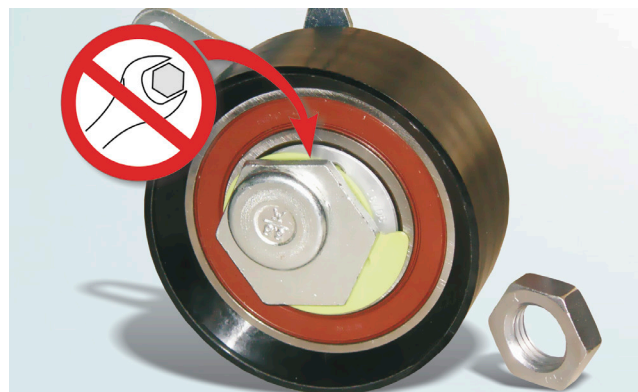
Снимка 2: Шестоъгълният фитинг на гърба на обтяжната ролка няма никаква функция
