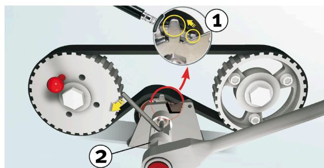
Снимка 1: Общ изглед на задвижването, на обтяжната ролка и на специализирания инструмент
