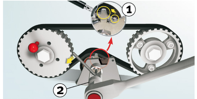
Kuva 1: Ruiskutuspumpun käyttöhihnajärjestelmä, hihnankiristin (tuotenro INA. 531 0573 30) sekä erikoistyökalu
