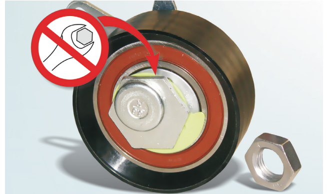
Kuva 2: Kiristimen takana olevalla levyllä ei ole toiminnallista merkitystä
