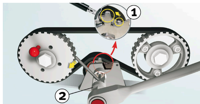
Figura 1: Privire de ansamblu asupra sistemului, rolei și a instrumentului special de montare
