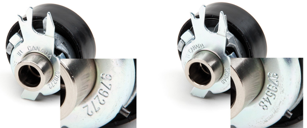
Kuva 2: Vasemmalla - kiristinpyörä 531 0252 30, oikealla - kiristinpyörä 531 0525 30
