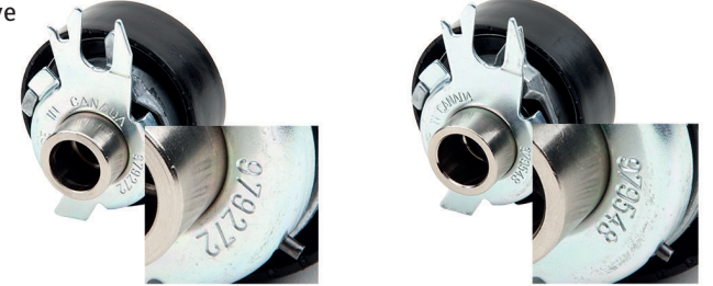
Şekil 2: Sağ - Gergi Rulmanı 531 0252 30, Sağ - Gergi Rulmanı 531 0525 30
