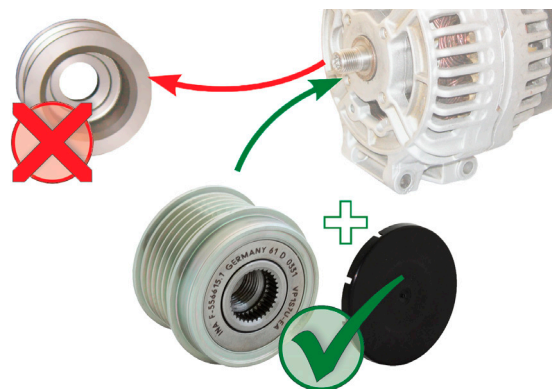
Снимка 1: Смяна на твърда ремъчна шайба с механизъм за свободен ход на генератор
