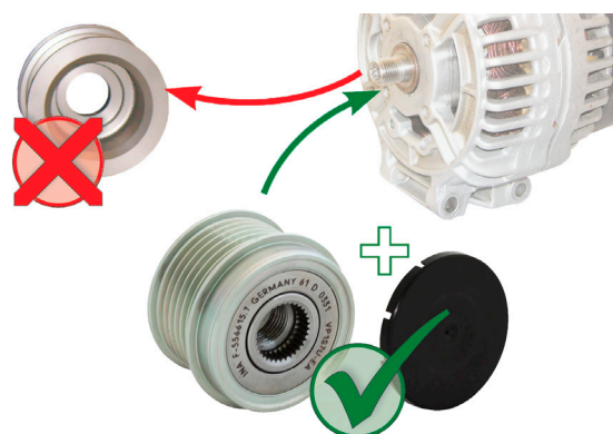
Obrázek 1: Výměna pevné řemenice za alternátorovou volnoběžku
