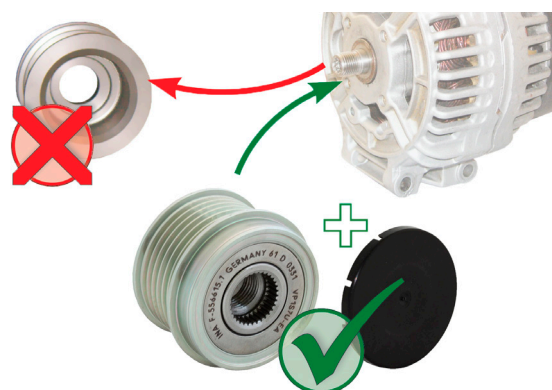
Billede 1: Udskiftning af en fast remskive for et friløbshjul til generator
