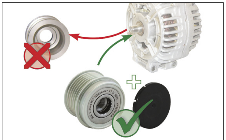
Fig. 1: Vervanging van starre rol door een dynamovrijlooprol
