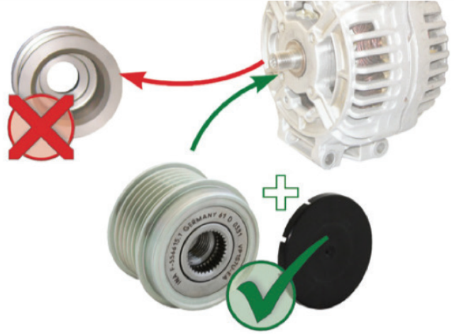
Resim 1: Rijit kasnağın devir ayarlı alternatör kasnağına değiştirilmesi
