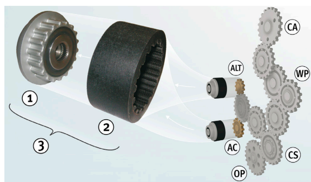
Obrázek 1: Alternátorová volnoběžka s flexibilní spojovací objímkou a pohonem koly s čelním ozubením
