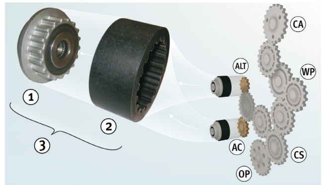
Kuva 1: Laturin vapaapyörä joustavalla liitosholkilla ja lieriöhammaspyörävedolla
