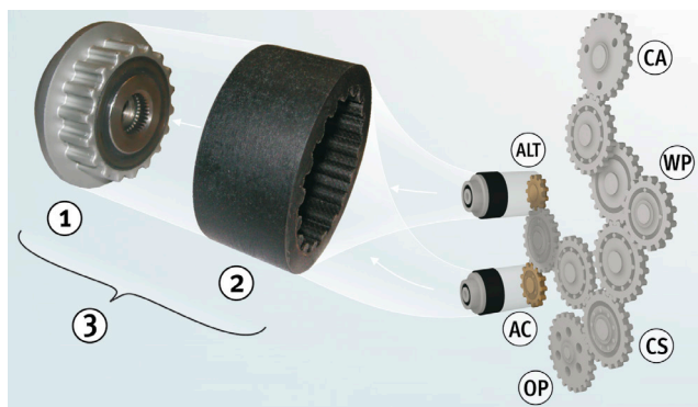
1. ábra: Generátor-szabardonfutó rugalmas kuplungaggal és homlokkerekes meghajtással
