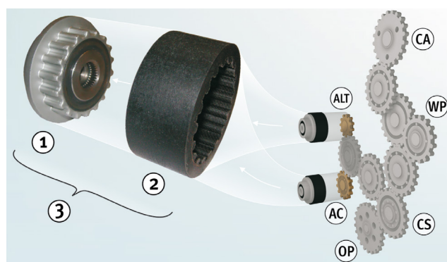
Bild 1: Generatorfrinav med flexibel kopplingsmuff och drivning genom främre kuggjul.
