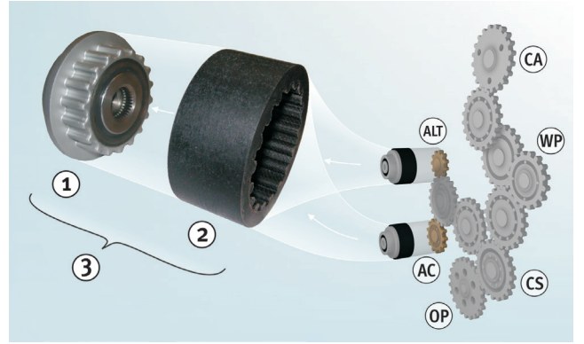
Şekil 1 : Esnek kaplin maşonu ve düz dişli tahriki ile devir ayarlı alternatör kasnağı
