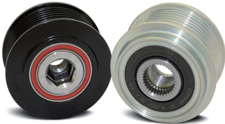
Şekil 2 : Devir ayarlı alternatör kasnağı 535 0229 10
