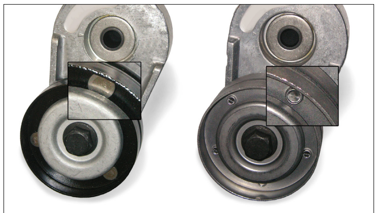
Slika 1: Detaljni izgled prethodne izvedbe remenice (lijevo) i nove izvedbe remenice (desno)
