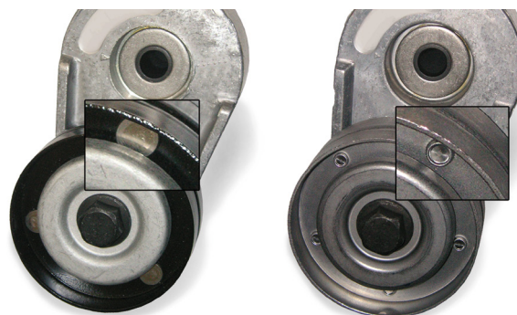
Figur 1: Detaljert visning over rullene i den tidligere utformingen (venstre) og den nye utformingen (høyre)
