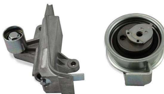
Obrázek 1: Dosavadní provedení, vlevo tlumič vibrací 533 0028 20, vpravo napínací kladka 531 0531 20
