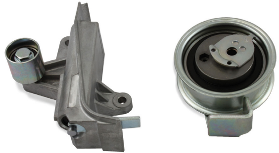
Kuva 1: Korvaantuva malli, vasemmalla värähtelynvaimennin 533 0028 20, oikealla kiristin 531 0531 20
