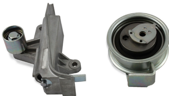
1. ábra: Balra az 533 0028 20 cikkszámú rezgéscsillapító, jobbra az 531 0531 20 cikkszámú feszítőgörgő
