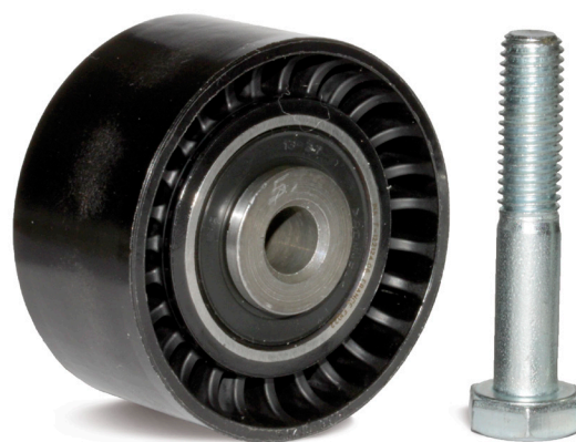
1. ábra: 532 0020 10 – INA műanyag terelőgörgő mellékelte rögzítőcsavarokkal
