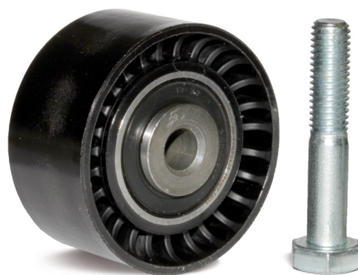
Figur 1: 532 0020 10 – INA styrerulle i plast med medfølgende festeskruer
