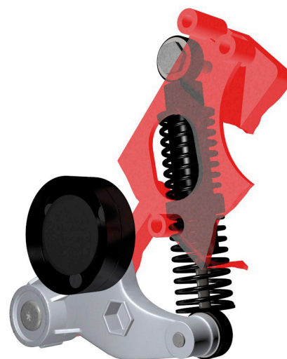
Obrázek 1: Kompletní napínací jednotka
