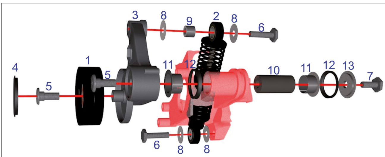
Obrázok 3: 533 0118 10 – INA - opravárenská súprava pre napínicu jednotku
