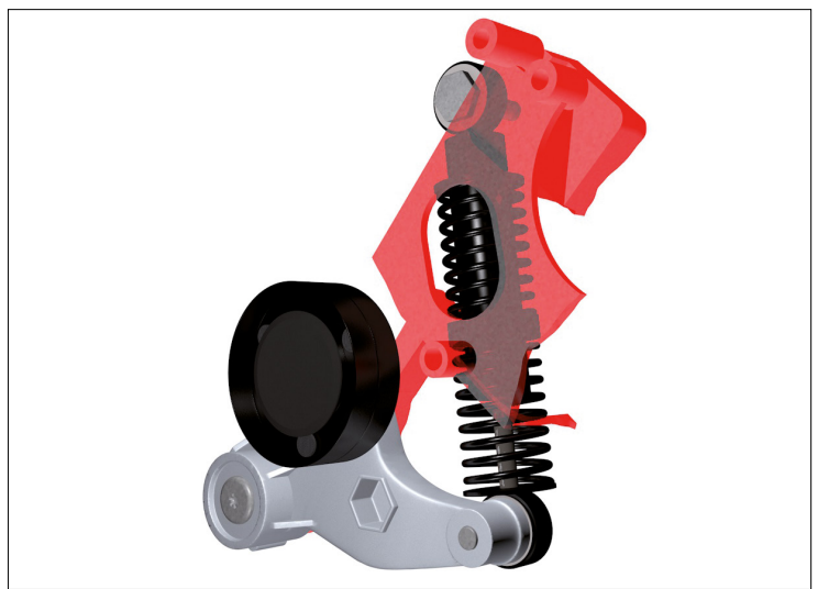
Obrázok 1: Kompletná napínicia jednotka
