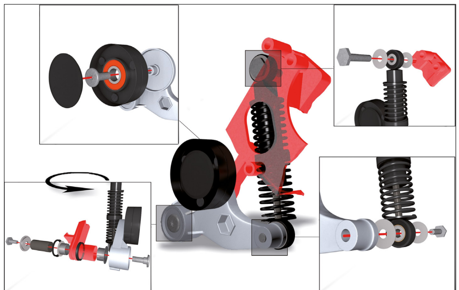
Obrázok 2: Prehľad upevňovacích dielov
