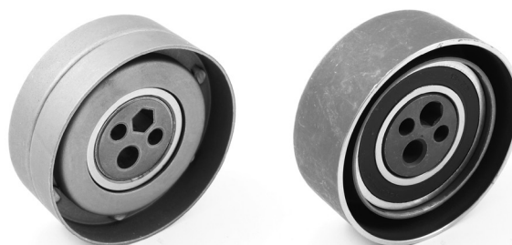
Рисунок 2: 531 0103 20 - Предыдущая конструкция (слева) и новая конструкция (справа)
